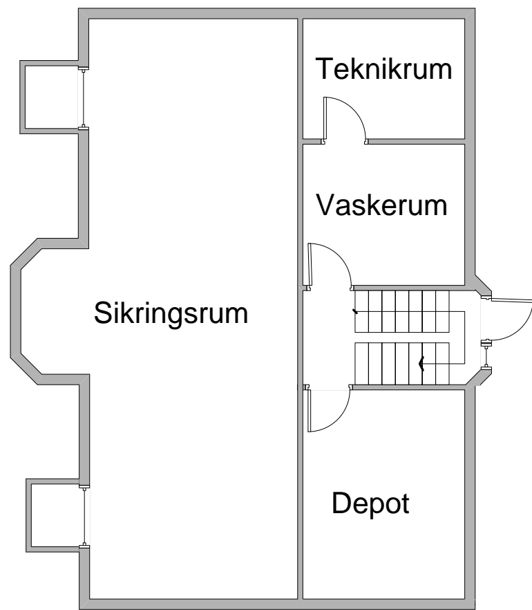
Kælderplan
